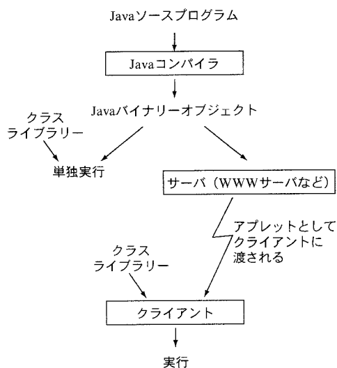
図1 Javaプログラム実行の流れ
