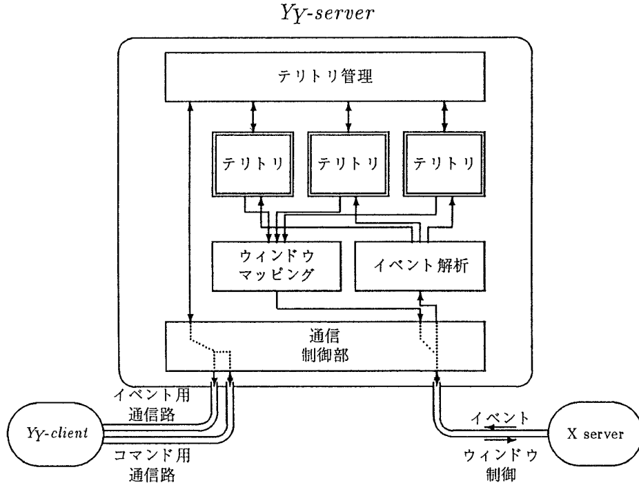
図 1: YyonX Version 1.0 における Yy-server の構成
