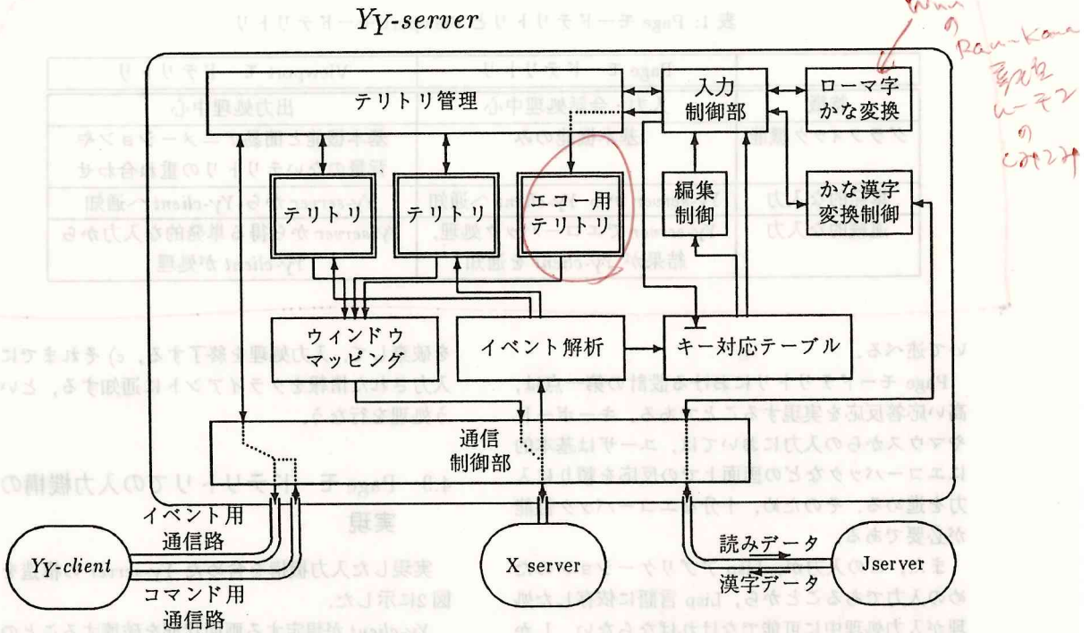
図 2: YyonX Version 1.2 における入力処理機構を含む Yy-server
